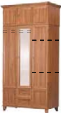
RGS83 szafa ubraniowa szer. / wys. / gł. 113 / 190 / 59 cm (122 / 195 / 63) cm
